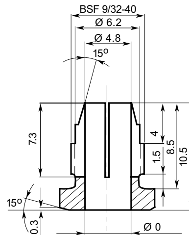
Spannzangen für 5,0-mm-Aufnahmen (Gewinde BSF 9/32 -40)
