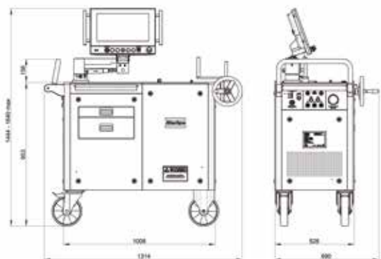
STbench Standard - kleiner Rahmen
