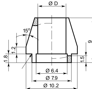
Spannzangen für 6,6-mm-Aufnahmen
