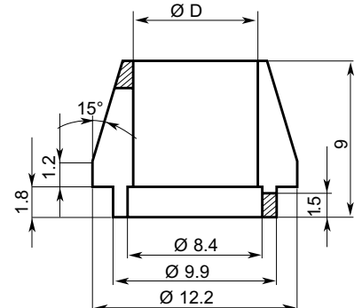
Spannzangen für 8,0-mm-Aufnahmen
